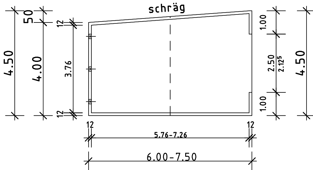
Grundriss
