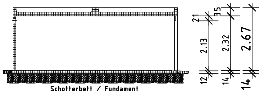
Schnitt
