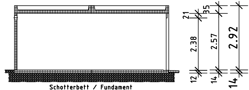
Schnitt
