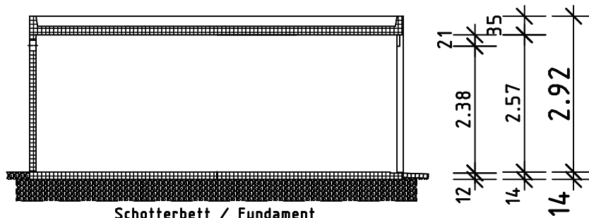
Schnitt
