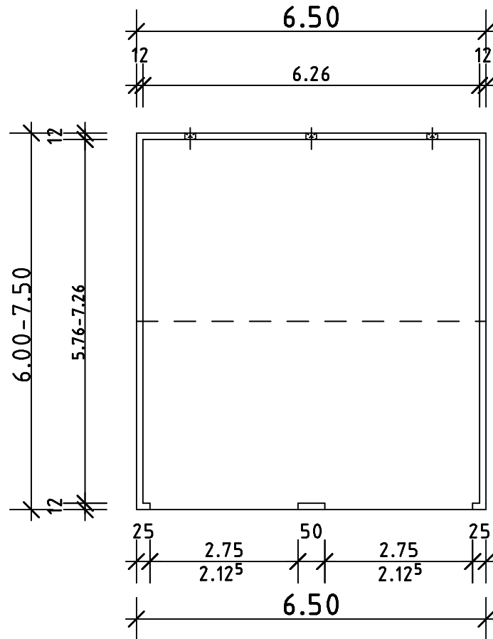
Grundriss
