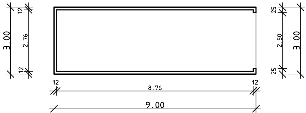
Grundriß
