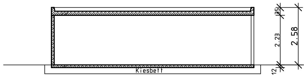
Schnitt
